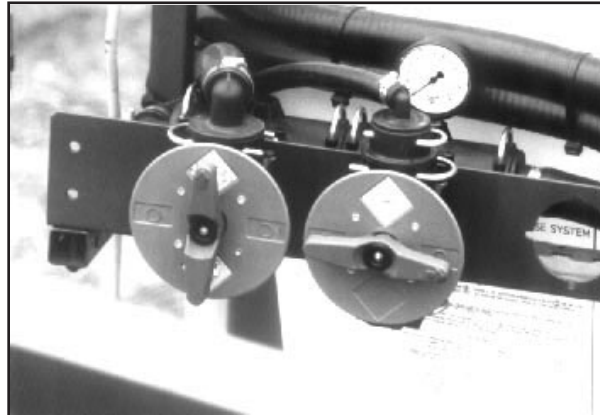
Fig. 55 Rinse Valve & Gauge
