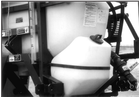
Fig. 54 Flush & Rinse Tank 2 (22 GAL.)
